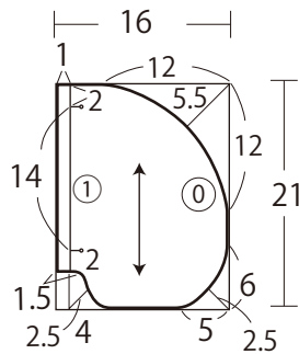
【ポケット】
